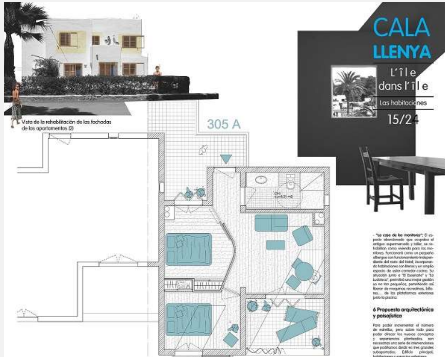
Detalle habitación 305 Bloque A P2 escala 1:50 Caja óptica de intervención. Habitación familiar para 4-6 personas.
